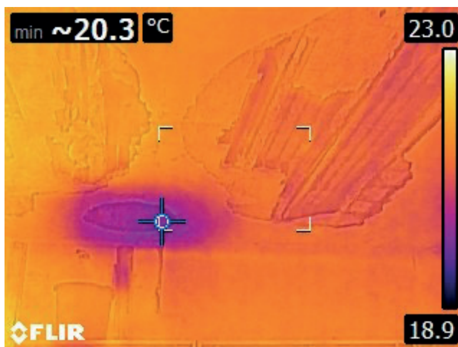
Esempio di ricerca ed individuazione delle porzioni sfondellate dell'intradosso di un solaio in latero-cemento.
